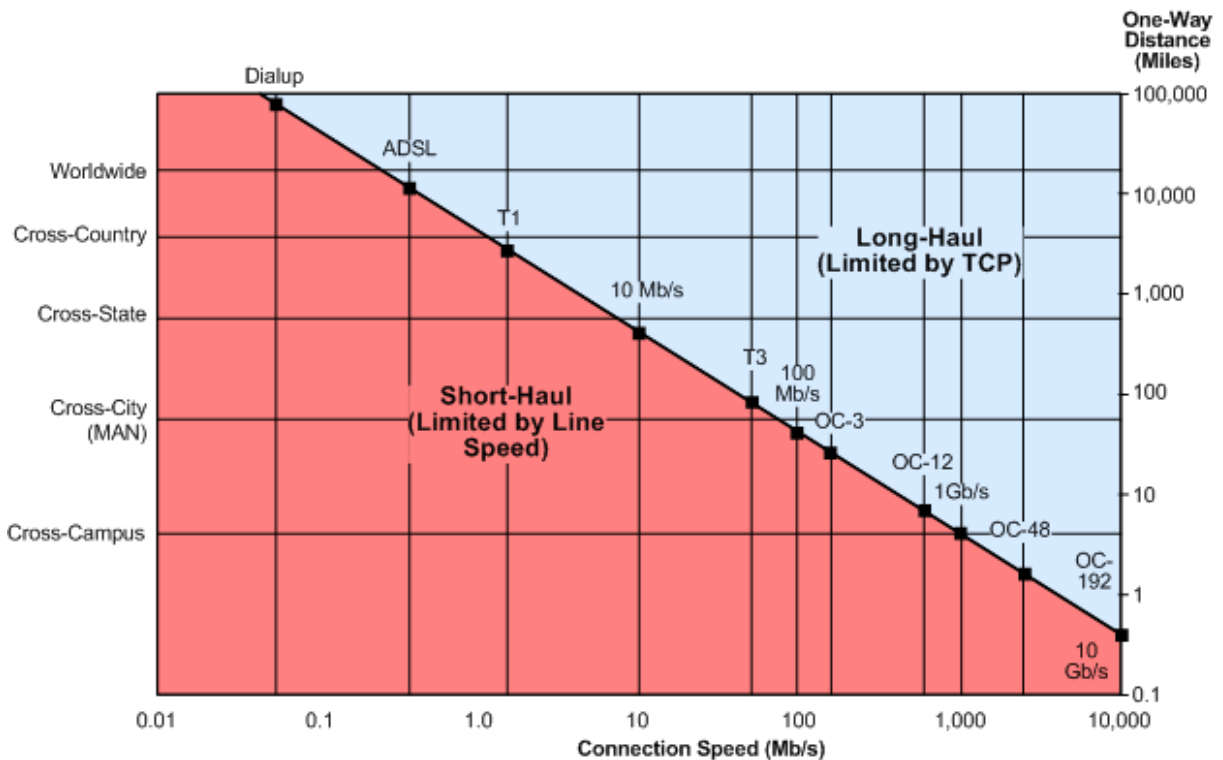
Ilustración 1. El rendimiento TCP no acelerado se desploma con la distancia
