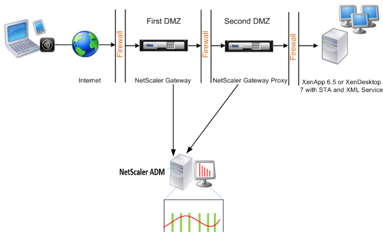
Figure 3. Citrix ADM déployé en mode double saut
