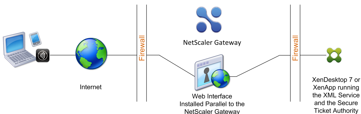
Figure 1. L'interface Web installée en parallèle à Citrix Gateway
