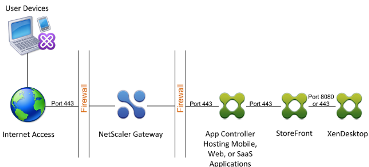
Figure 1. Déploiement de Citrix Gateway avec Endpoint Management devant StoreFront
