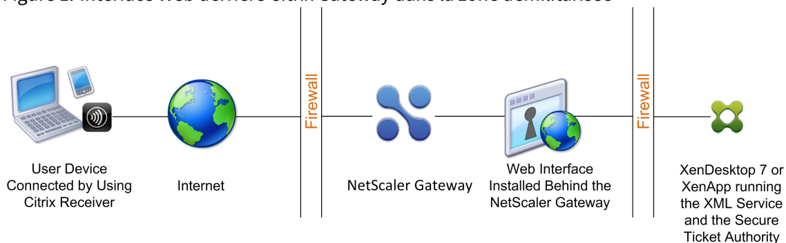
Figure 1. Interface Web derrière Citrix Gateway dans la zone démilitarisée
