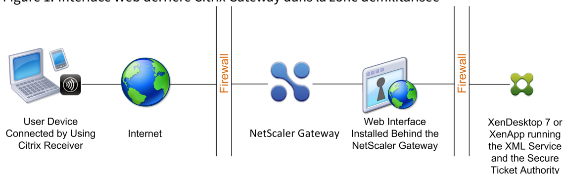
Figure 1. Interface Web derrière Citrix Gateway dans la zone démilitarisée
