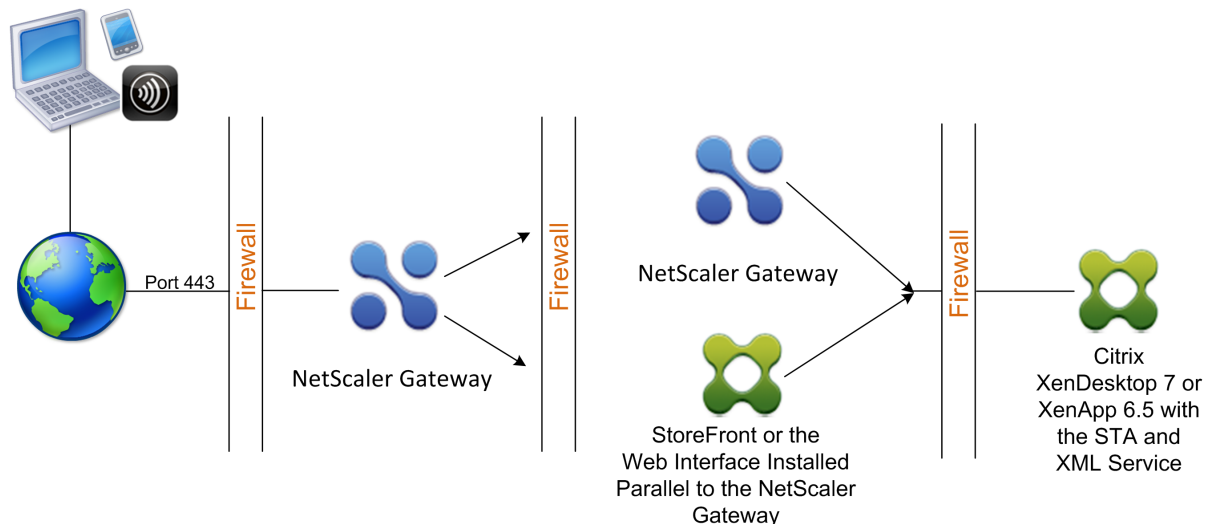
図 1: ダブルホップ DMZ に展開された NetScaler Gateway アプライアンス
