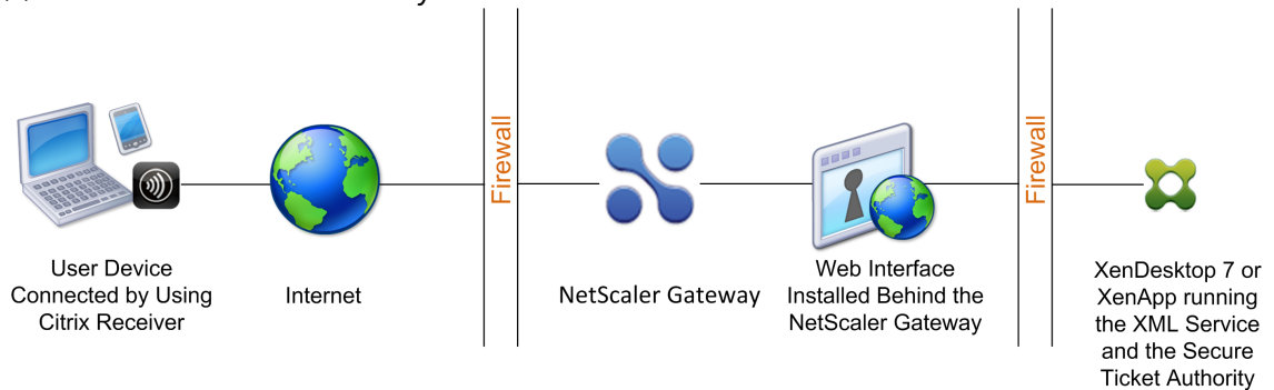
図 1: DMZ の NetScaler Gateway
