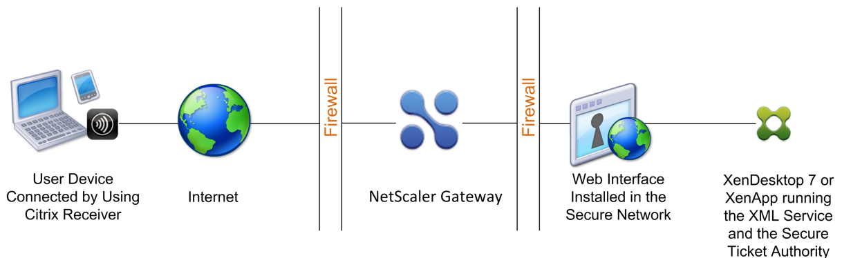
図 1: セキュアネットワーク内に配置された Web インターフェイス
