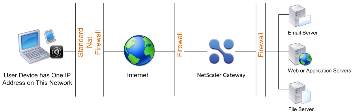
图 1. 通过两个内部防火墙与用户设备进行连接
