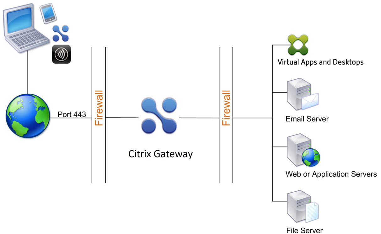
图 1. 在 DMZ 中部署的 Citrix Gateway
