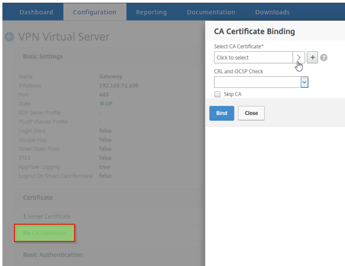
图 1. 为智能卡身份验证添加根证书
