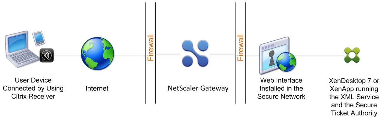
图 1. Web Interface 位于安全网络内
