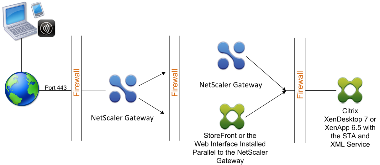
图 1. 在双跃点 DMZ 中部署的 Citrix Gateway 设备
