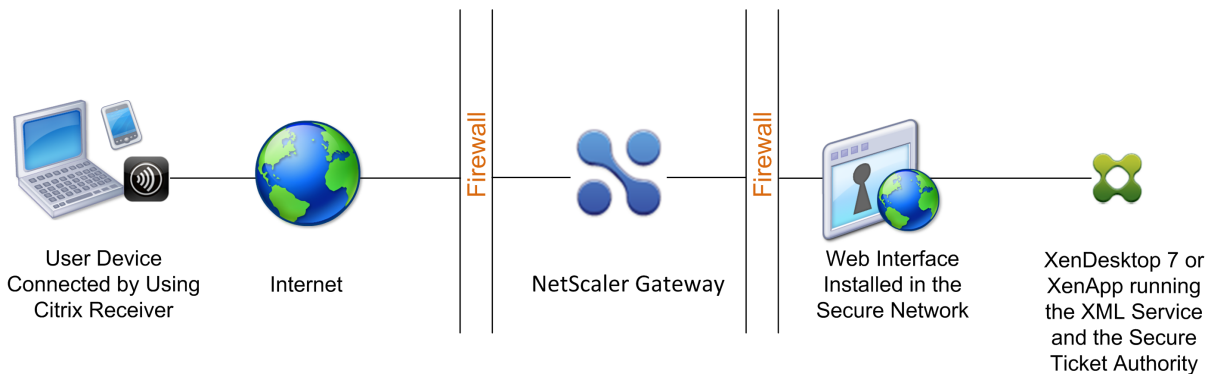
图 1. Web Interface 位于安全网络内
