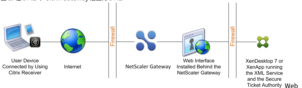
图 1. 在 DMZ 中 Citrix Gateway 后面的 DMZ
