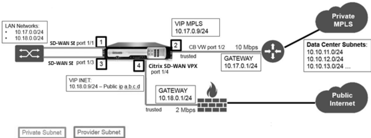
方案 2. 分支拓扑：内联模式
